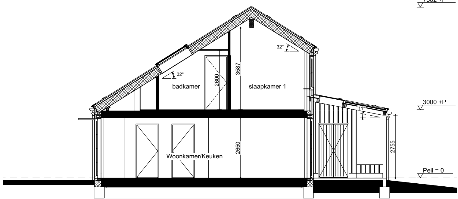
DOORSNEDE A-A
