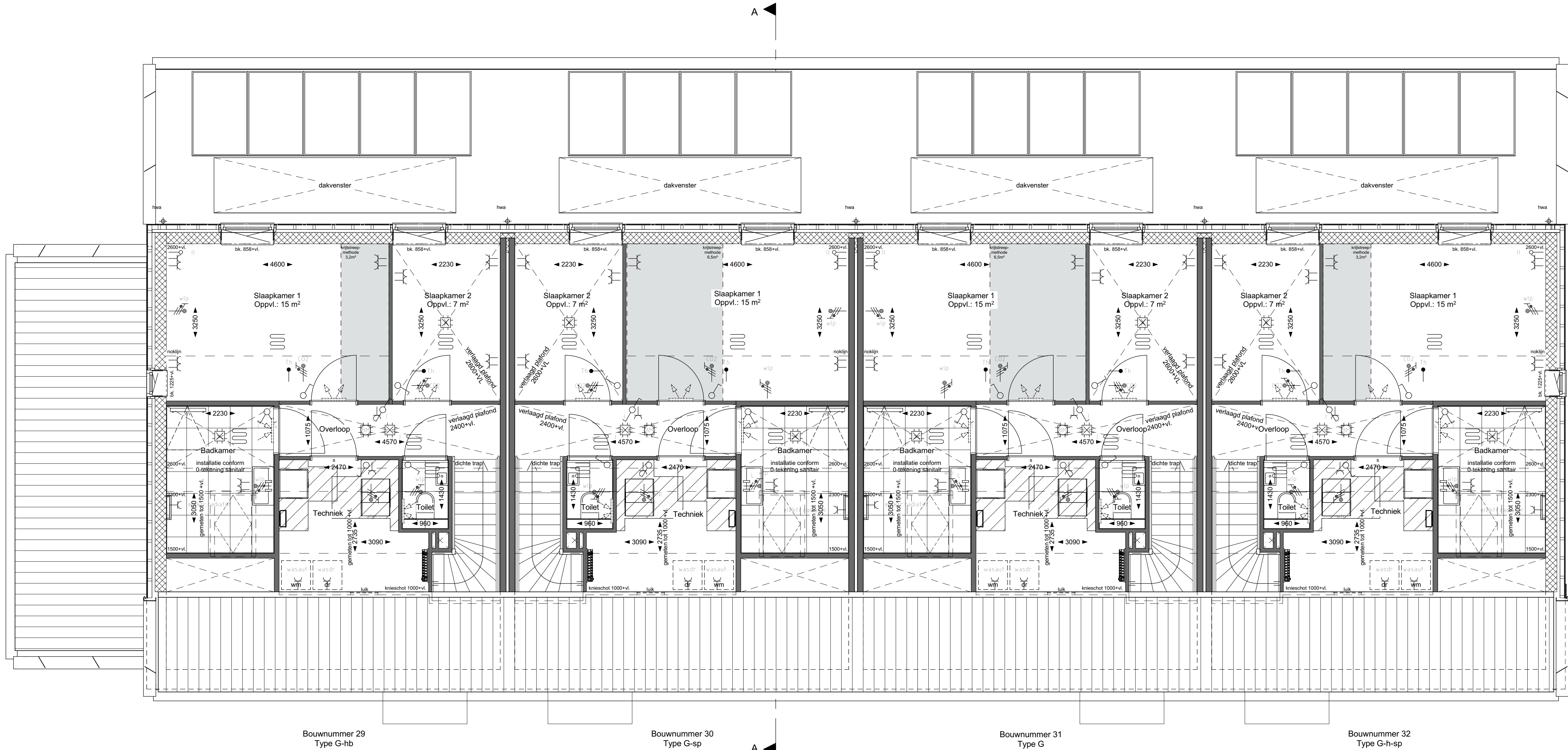
1e VERDIEPING
