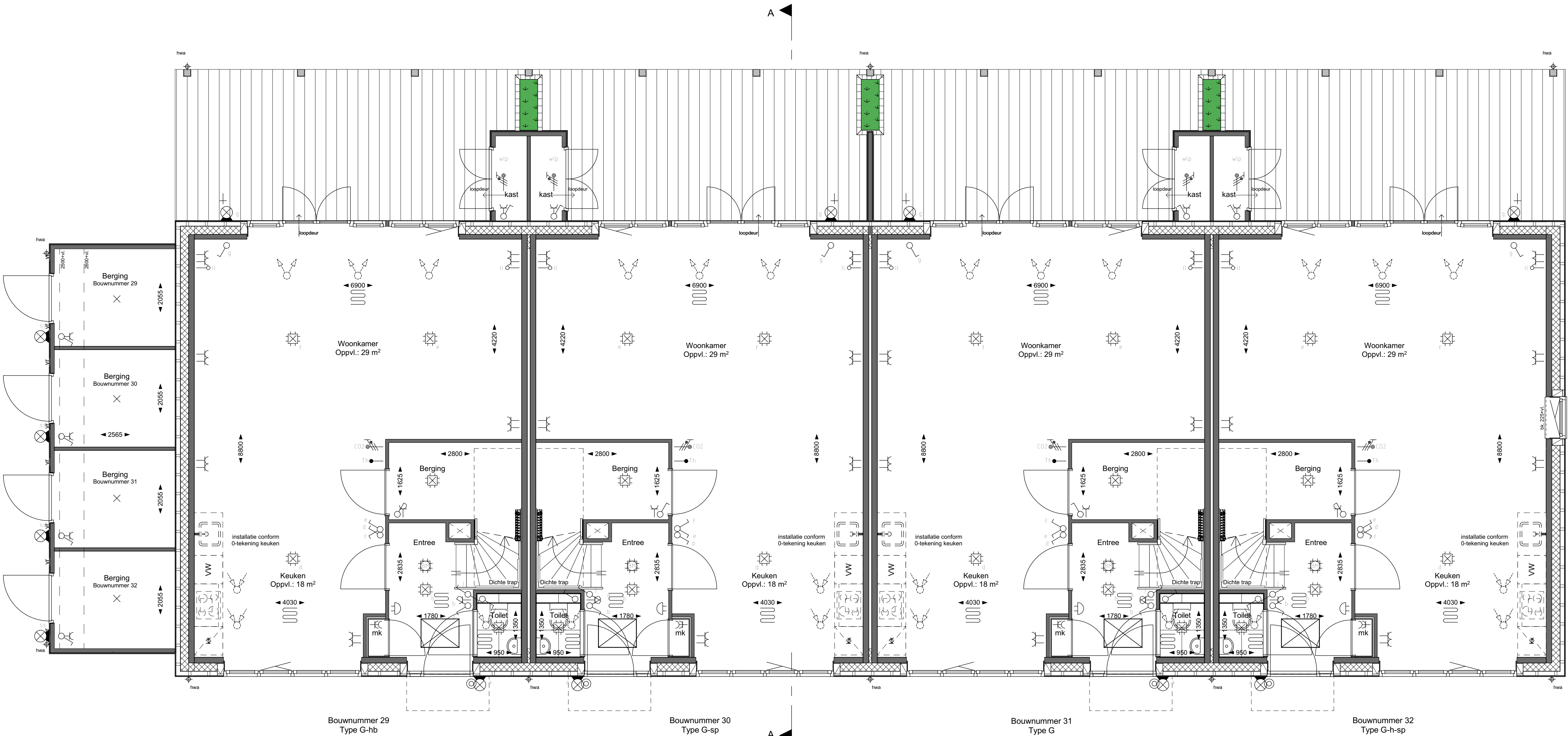
BEGANE GROND
